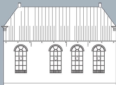
Noordgevel
