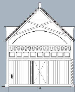
Dwarsdoorsnede
