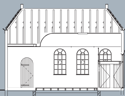
Langsdoorsnede
